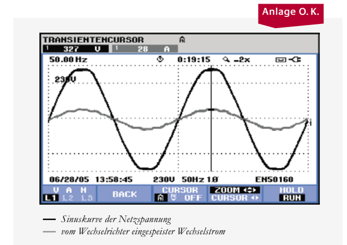
Wechselrichterüberprüfung
