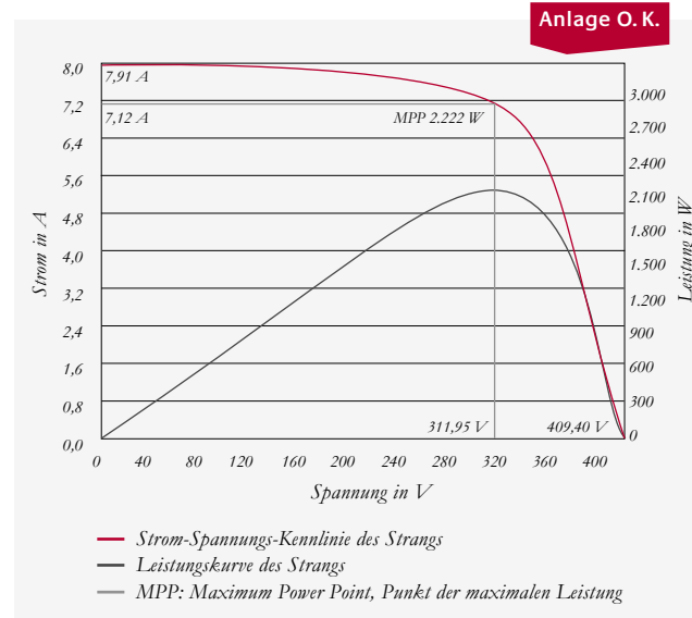
Kennlinienmessung
