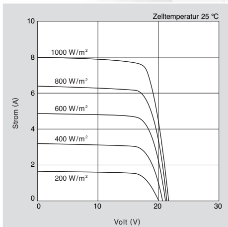
Strom-Spannungskennlinie des Moduls KC125GH-2 bei verschiedener Einstrahlung.
