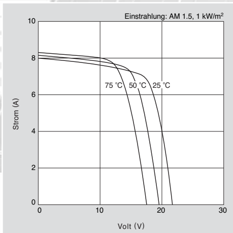
Strom-Spannungskennlinie des Moduls KC125GH-2 bei verschiedenen Zelltemperaturen.
