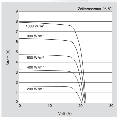
Strom-Spannungs-Kennlinie des Moduls KC125GHT-2 bei verschiedener Einstrahlung.
