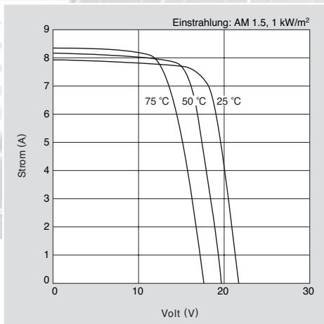
Strom-Spannungs-Kennlinie des Moduls KC125GHT-2 bei verschiedenen Zelltemperaturen.
