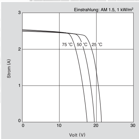
Strom-Spannungs-Kennlinie des Moduls KC40 bei verschiedenen Zelltemperaturen.
