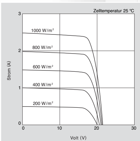
Strom-Spannungs-Kennlinie des Moduls KC40 bei verschiedener Einstrahlung.
